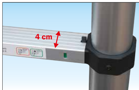
Gradini profondi 4 cm con superficie anti-scivolo dotato di indicatore colorato di conferma corretto bloccaggio
