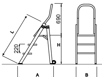
Spostamento a carriola con ruote Ø 80 mm in plastica rinforzata
